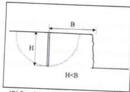
(D) Too large front burden
